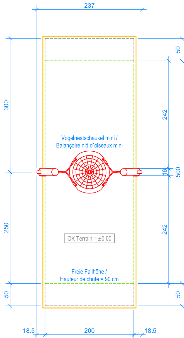
GRUNDRISS / PLAN 1:50
