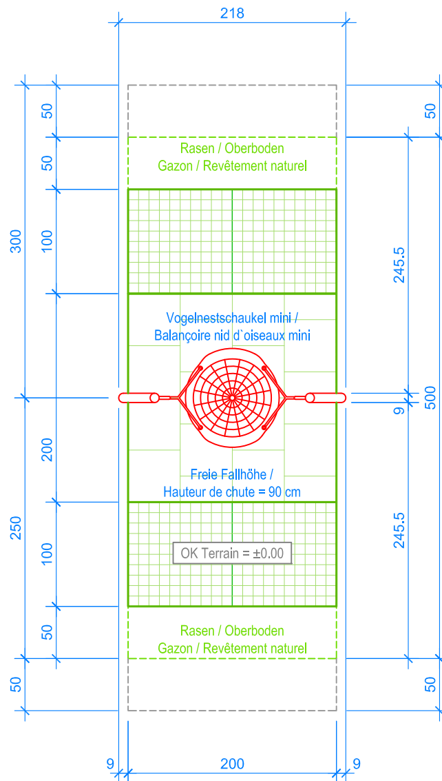
GRUNDRISS / PLAN 1:50
