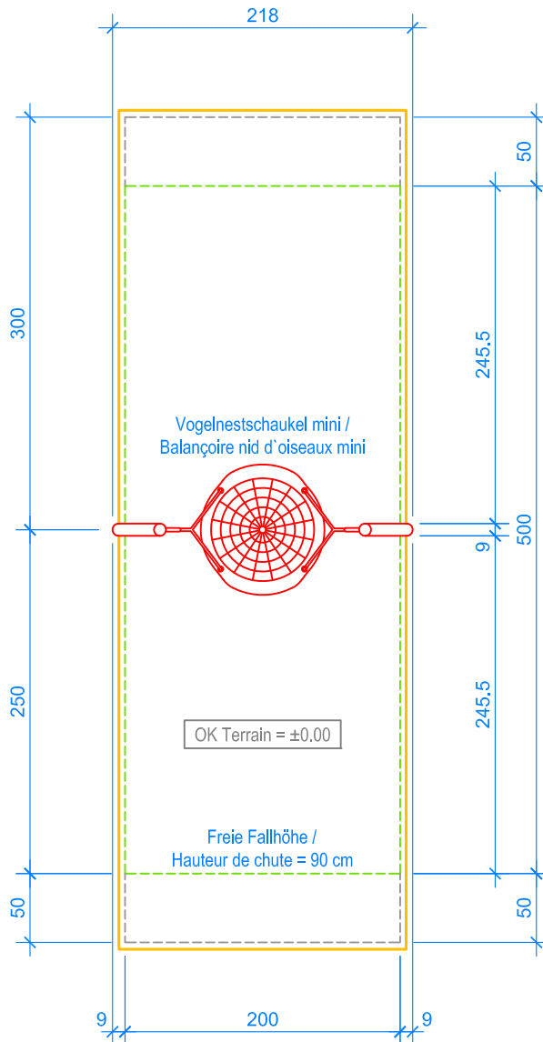
GRUNDRISS / PLAN 1:50
