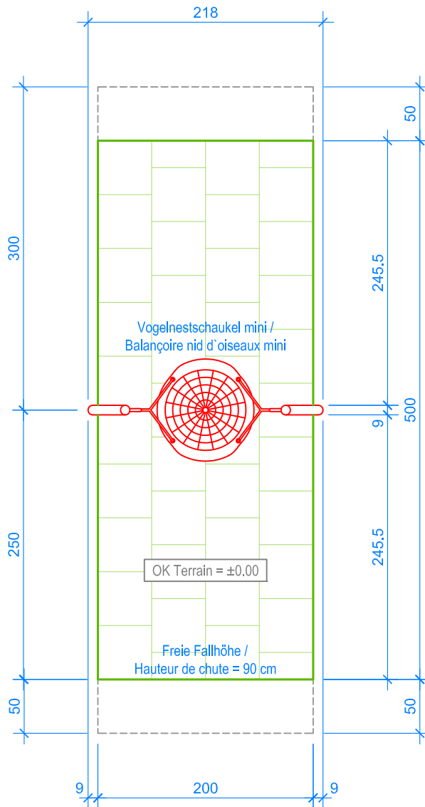
GRUNDRISS / PLAN 1:50
