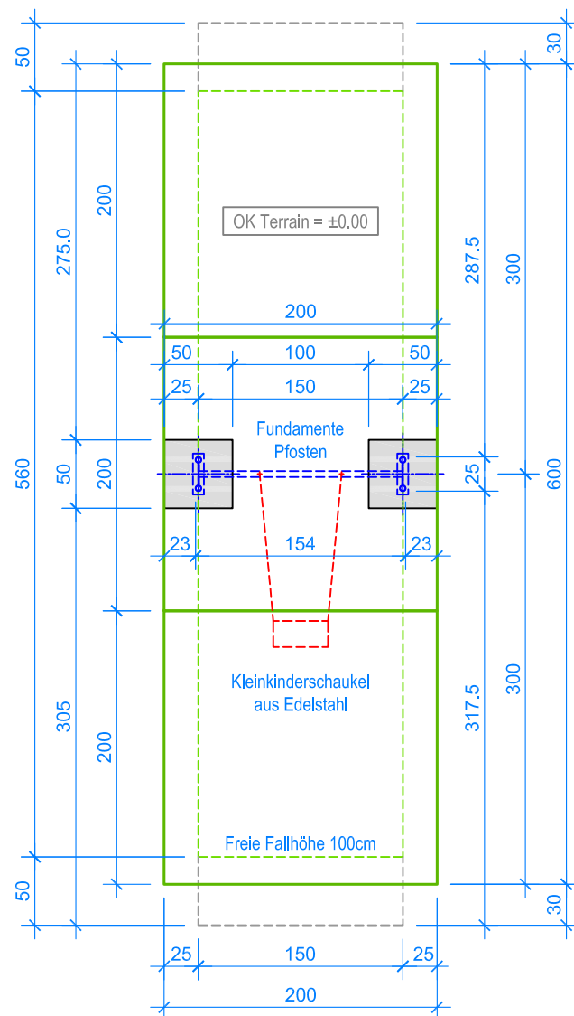
GRUNDRISS 1:50
