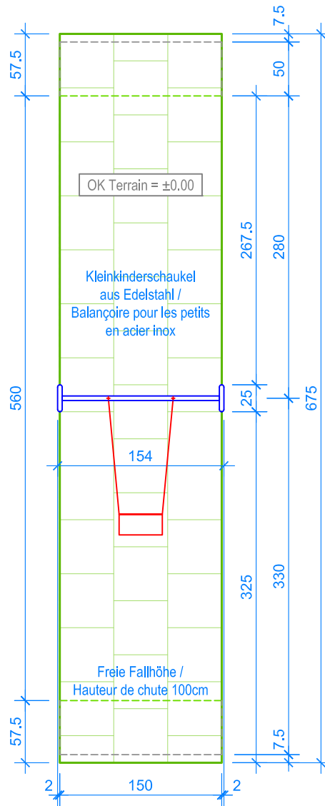
GRUNDRISS / PLAN 1:50
