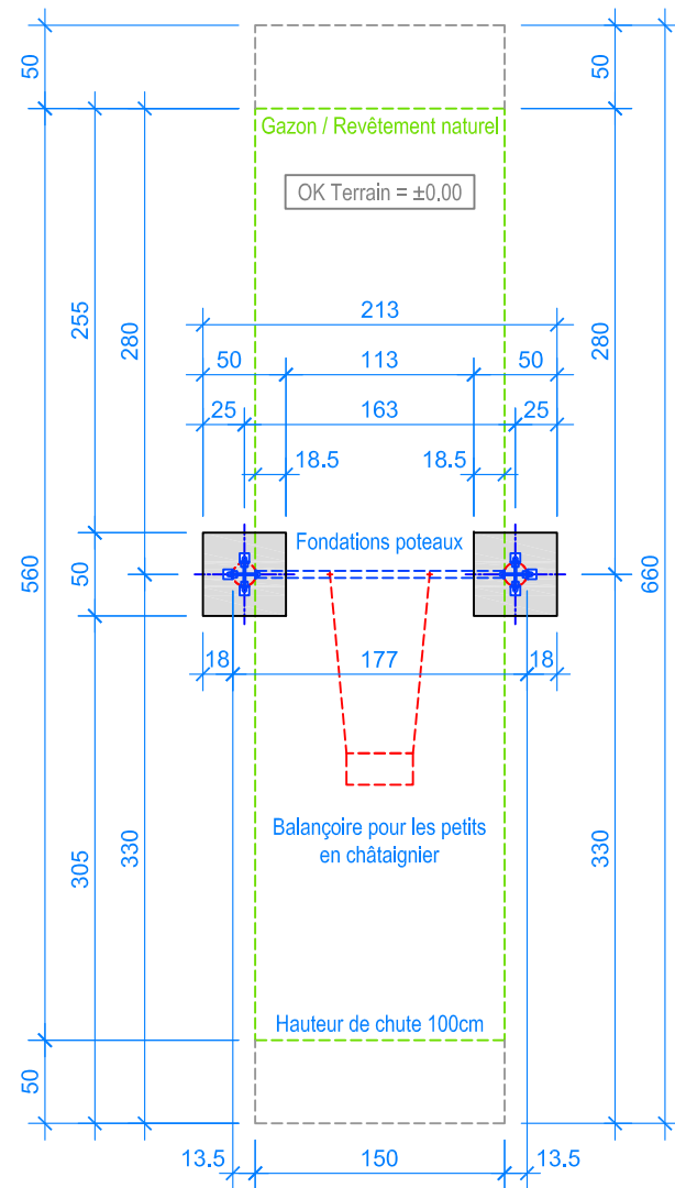
PLAN 1:50
