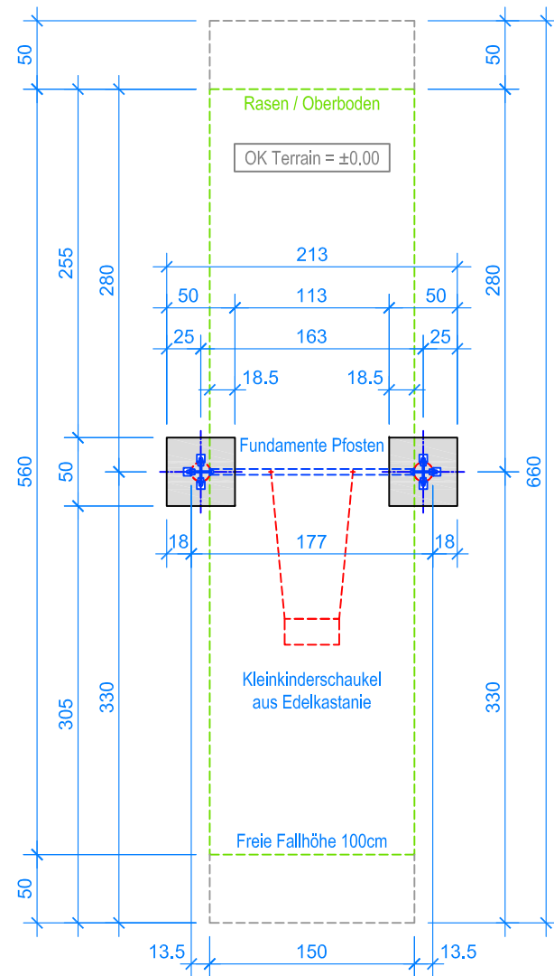
GRUNDRISS 1:50
