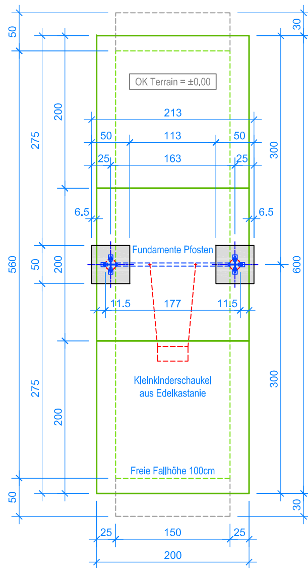
GRUNDRISS 1:50
