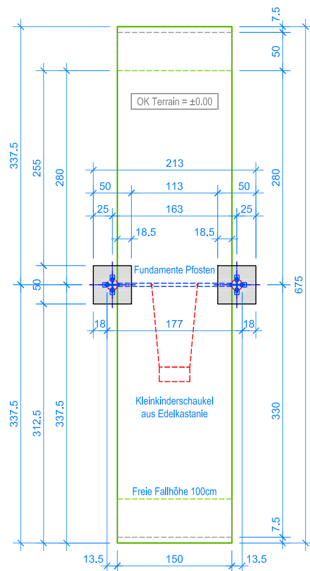
GRUNDRISS 1:50
