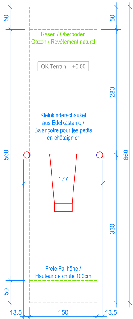
GRUNDRISS / PLAN 1:50
