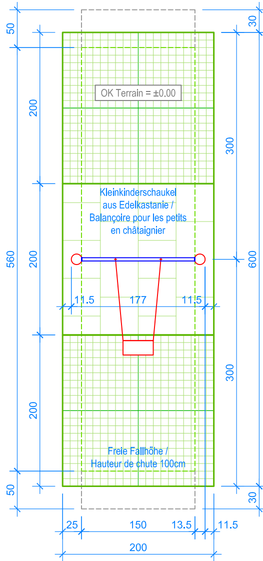
GRUNDRISS / PLAN 1:50
