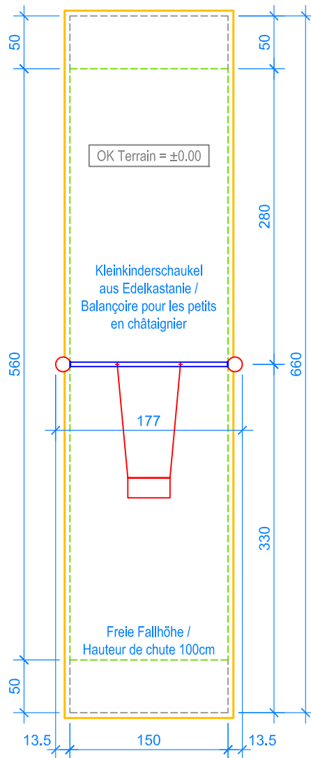
GRUNDRISS / PLAN 1:50
