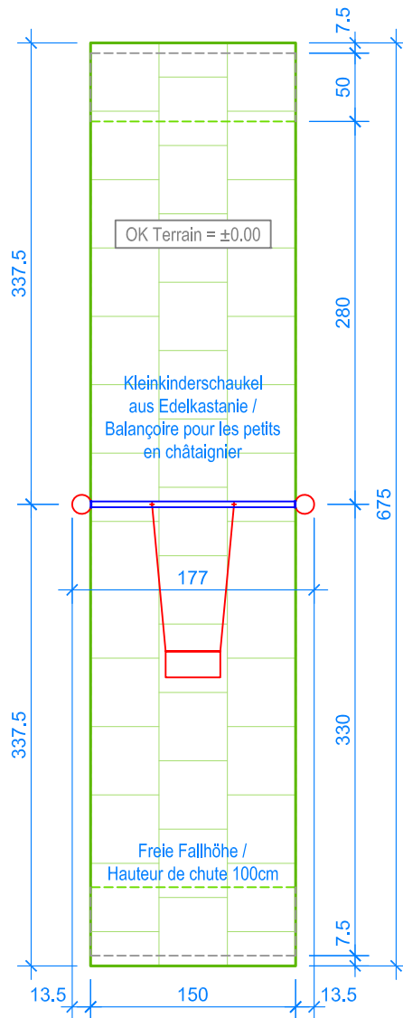
GRUNDRISS / PLAN 1:50
