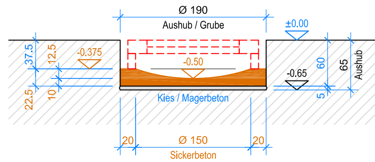
SCHNITT A-A 1:50
