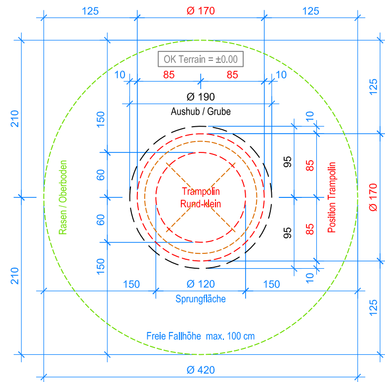
GRUNDRISS 1:50
