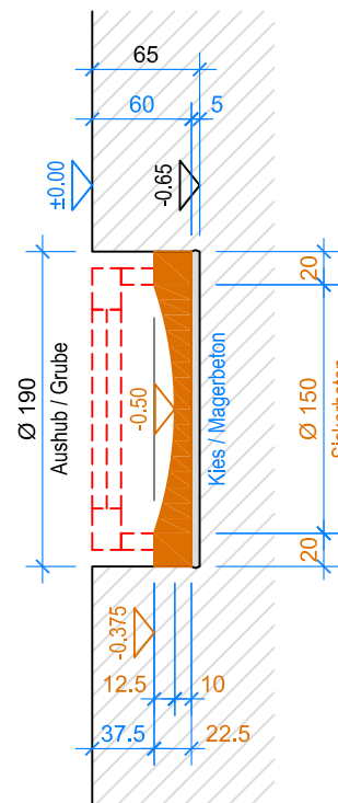
SCHNITT B-B 1:50
