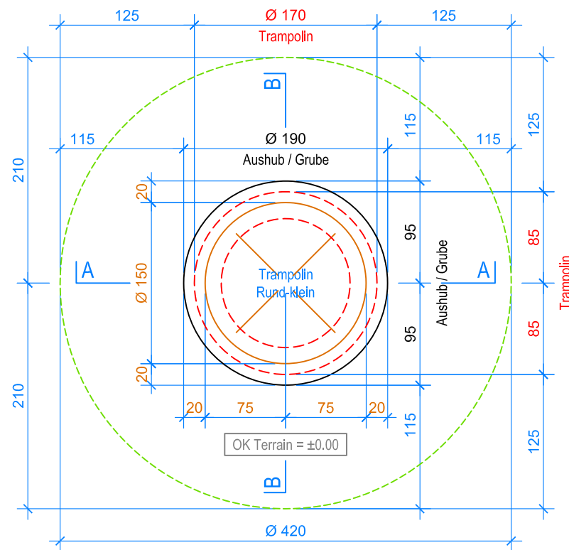
GRUNDRISS 1:50
