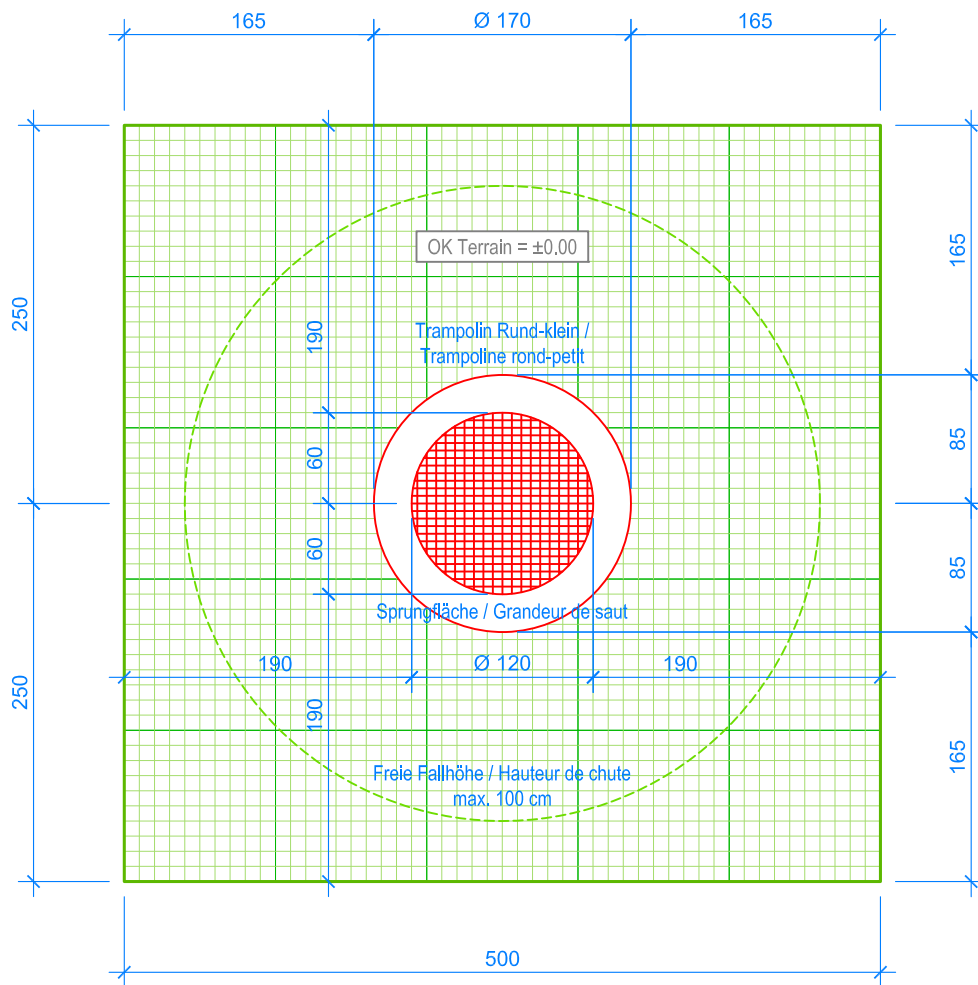
GRUNDRISS / PLAN 1:50
