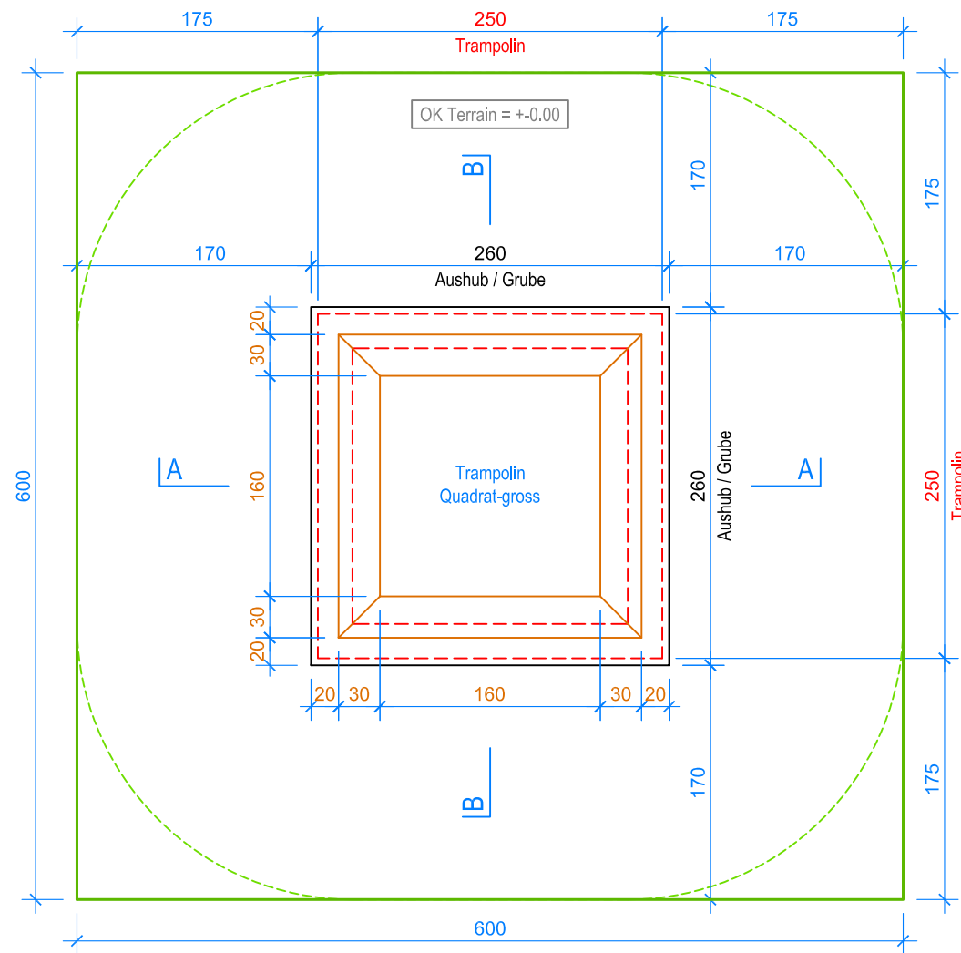
GRUNDRISS 1:50
