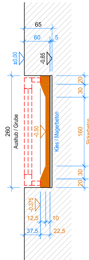
SCHNITT B-B 1:50
