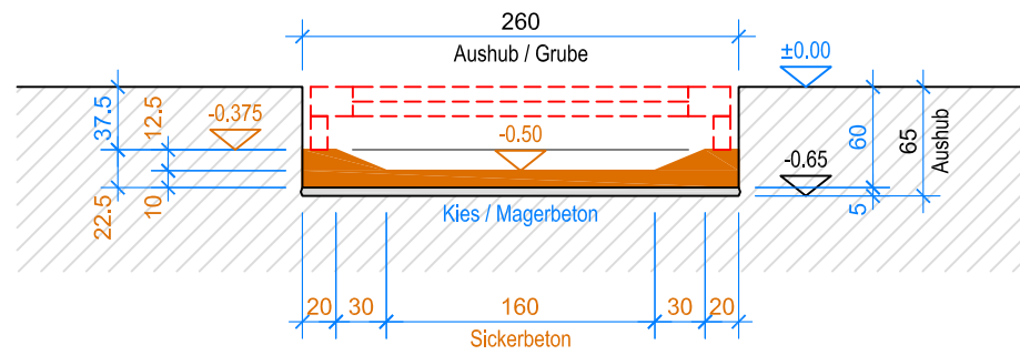
SCHNITT A-A 1:50
