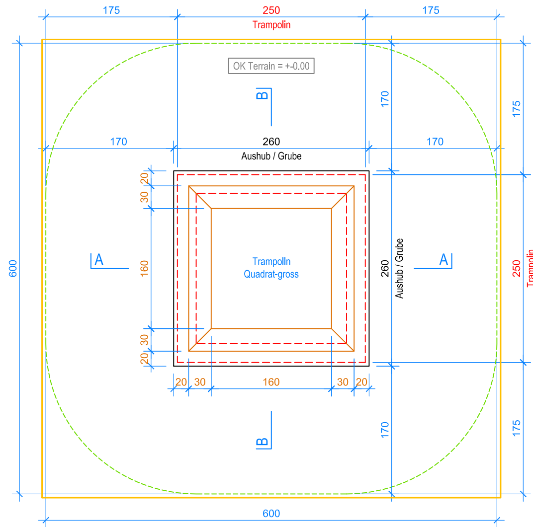
GRUNDRISS 1:50
