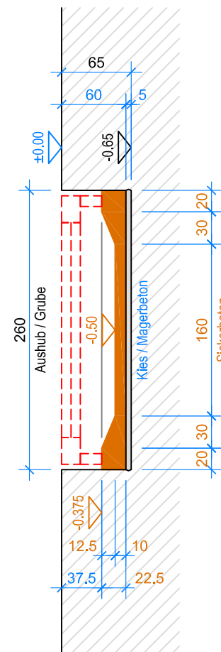
SCHNITT B-B 1:50
