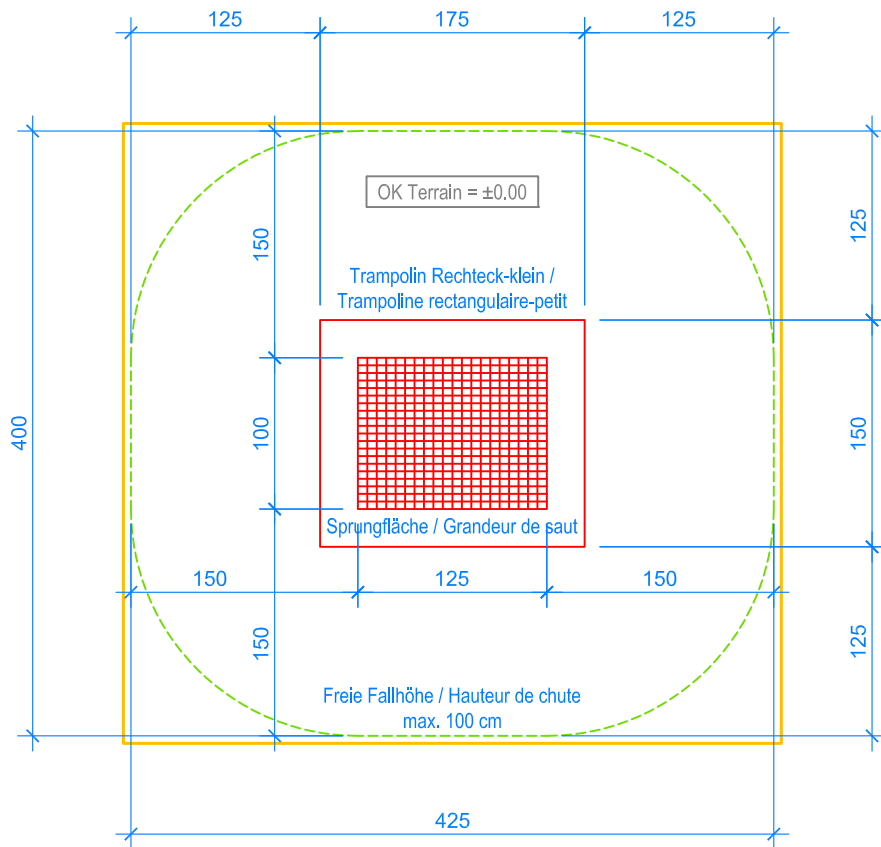
GRUNDRISS / PLAN 1:50
