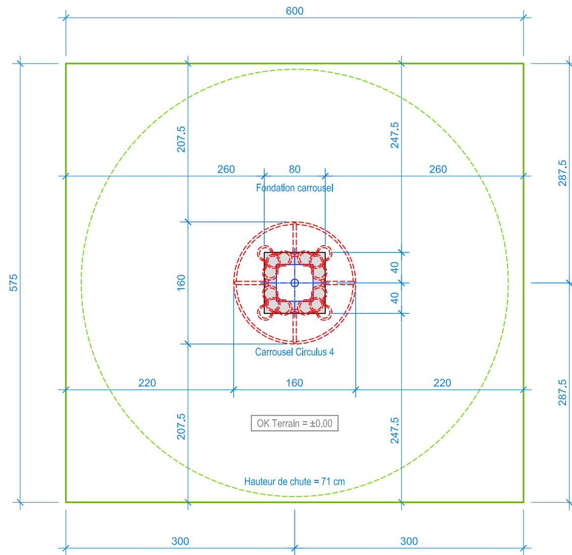
PLAN 1:50
