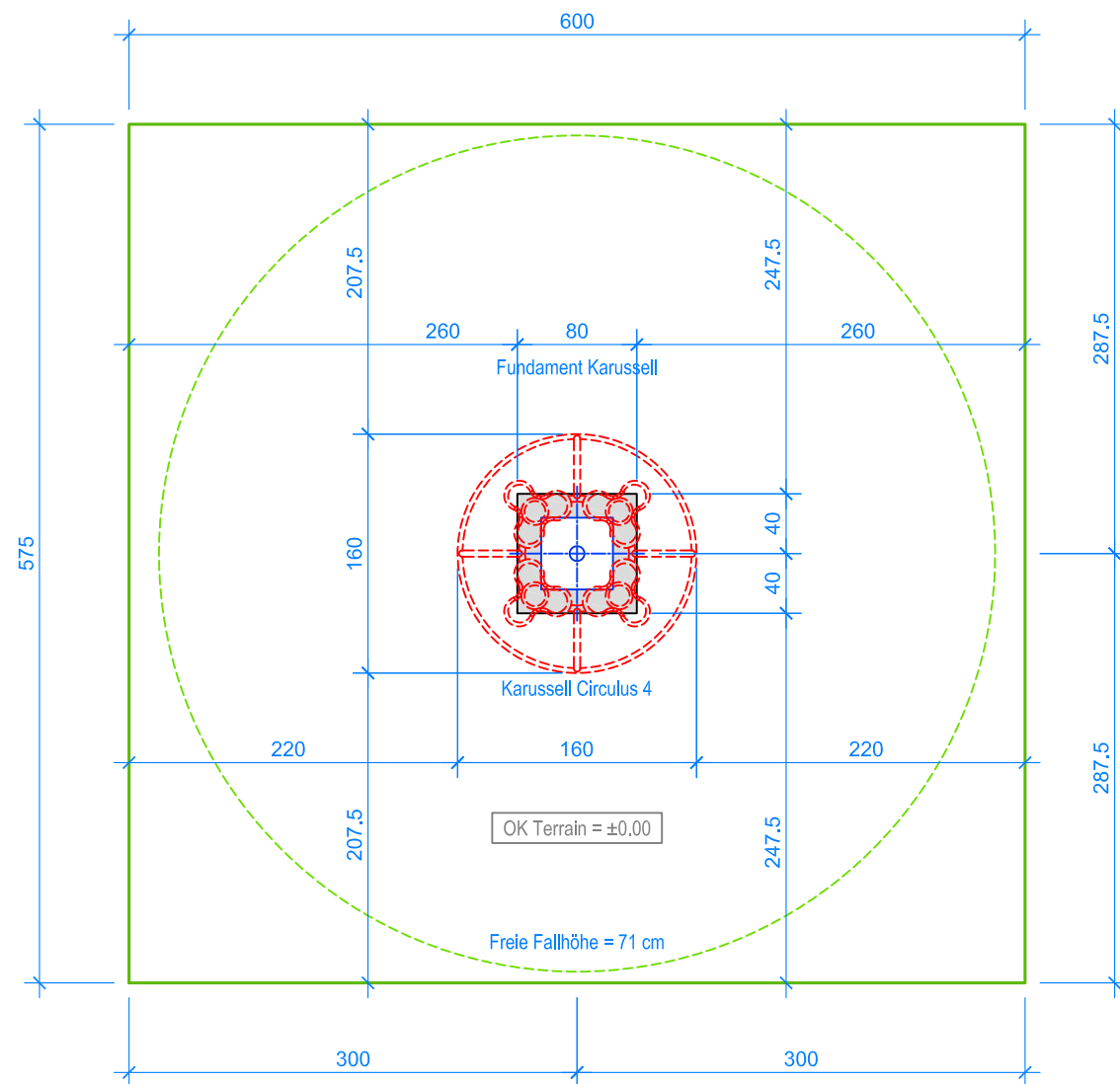
GRUNDRISS 1:50
