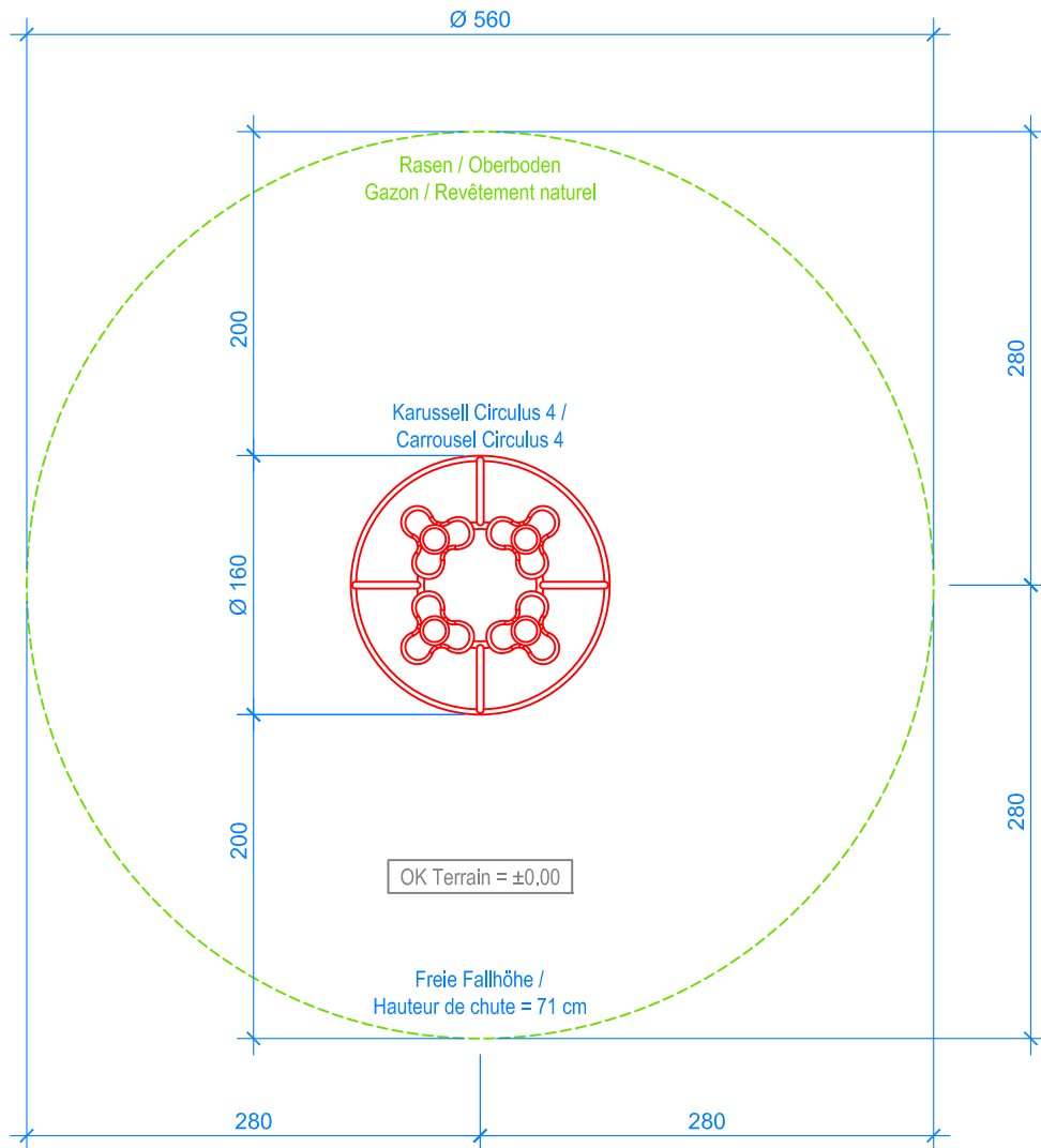
GRUNDRISS / PLAN 1:50
