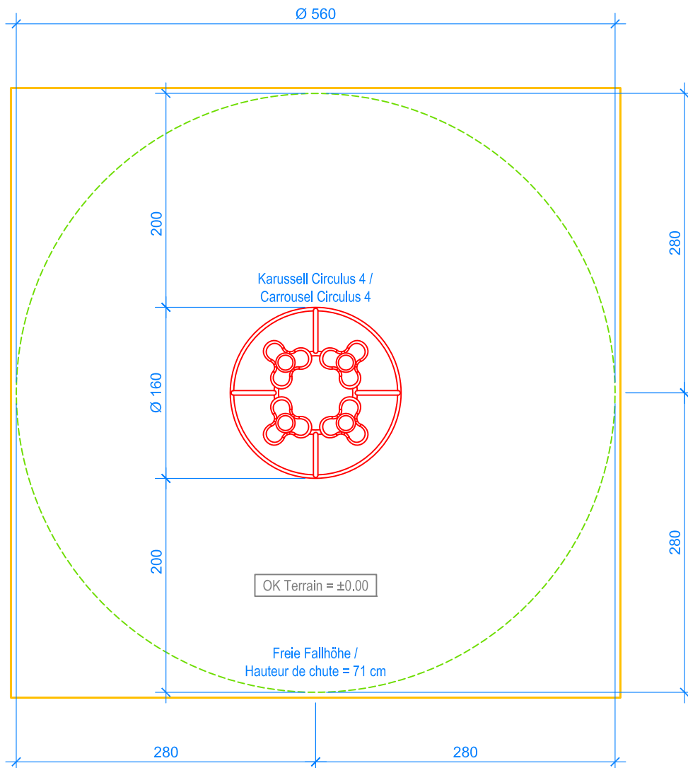
GRUNDRISS / PLAN 1:50
