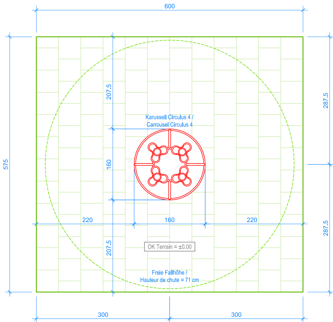
GRUNDRISS / PLAN 1:50
