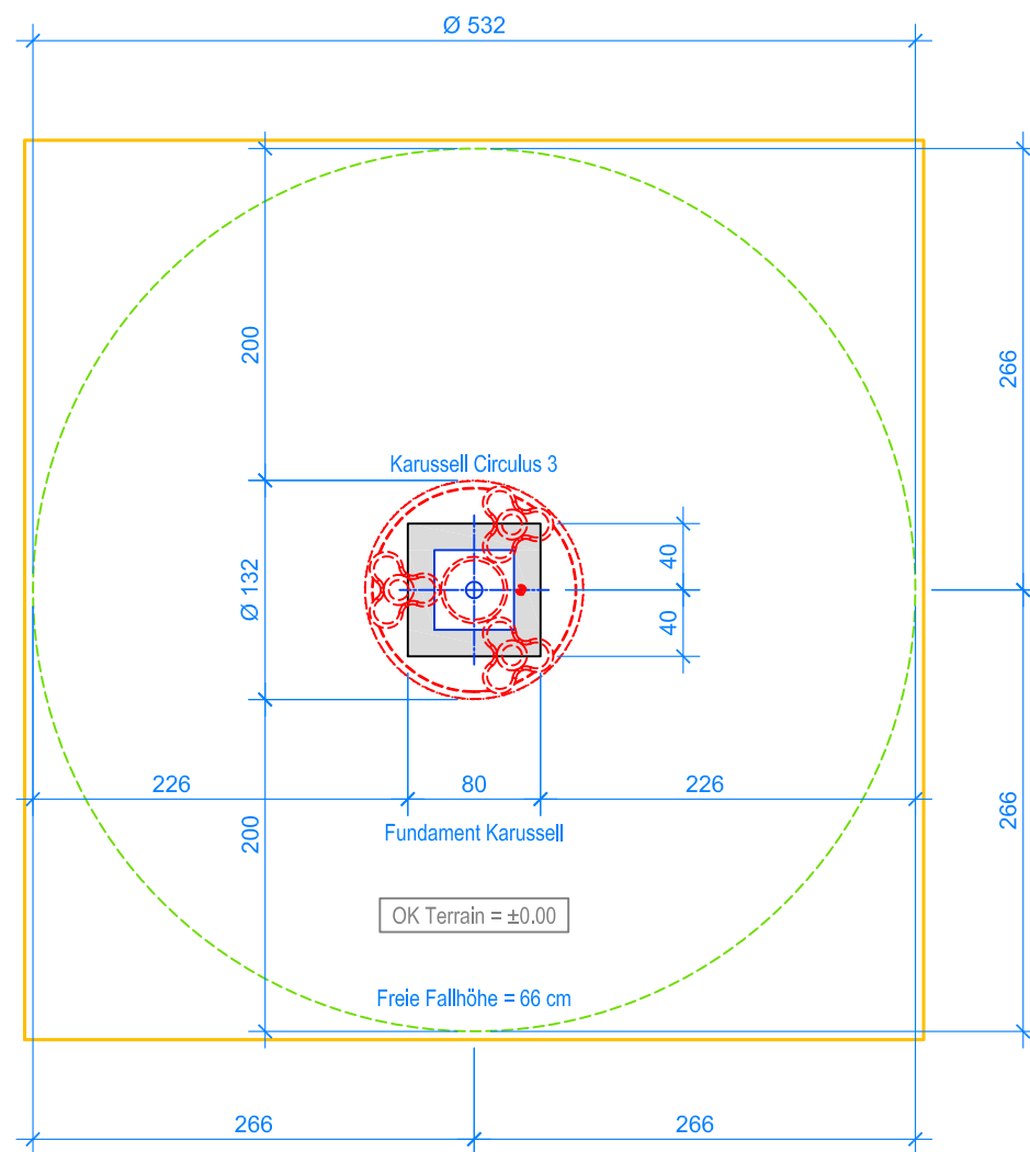
GRUNDRISS 1:50
