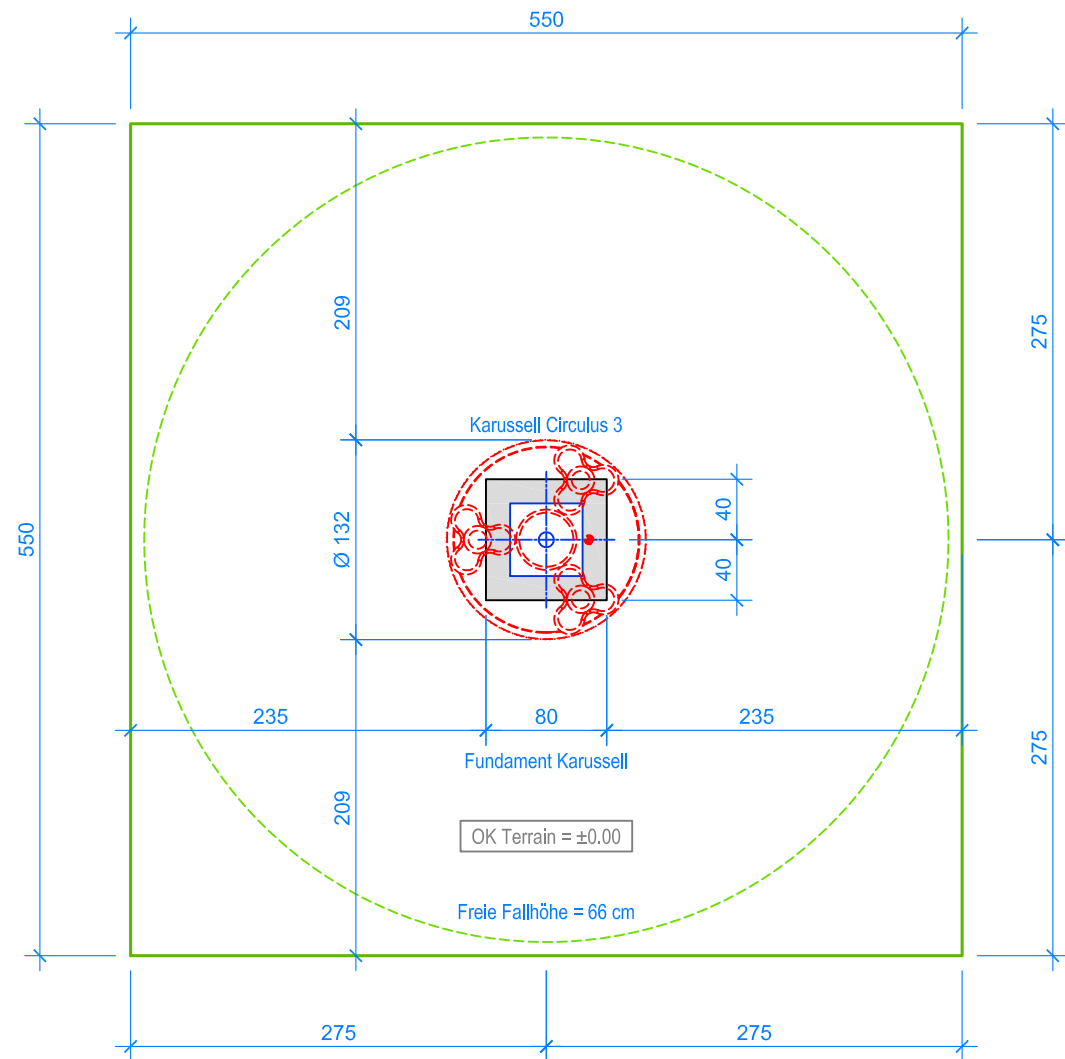
GRUNDRISS 1:50
