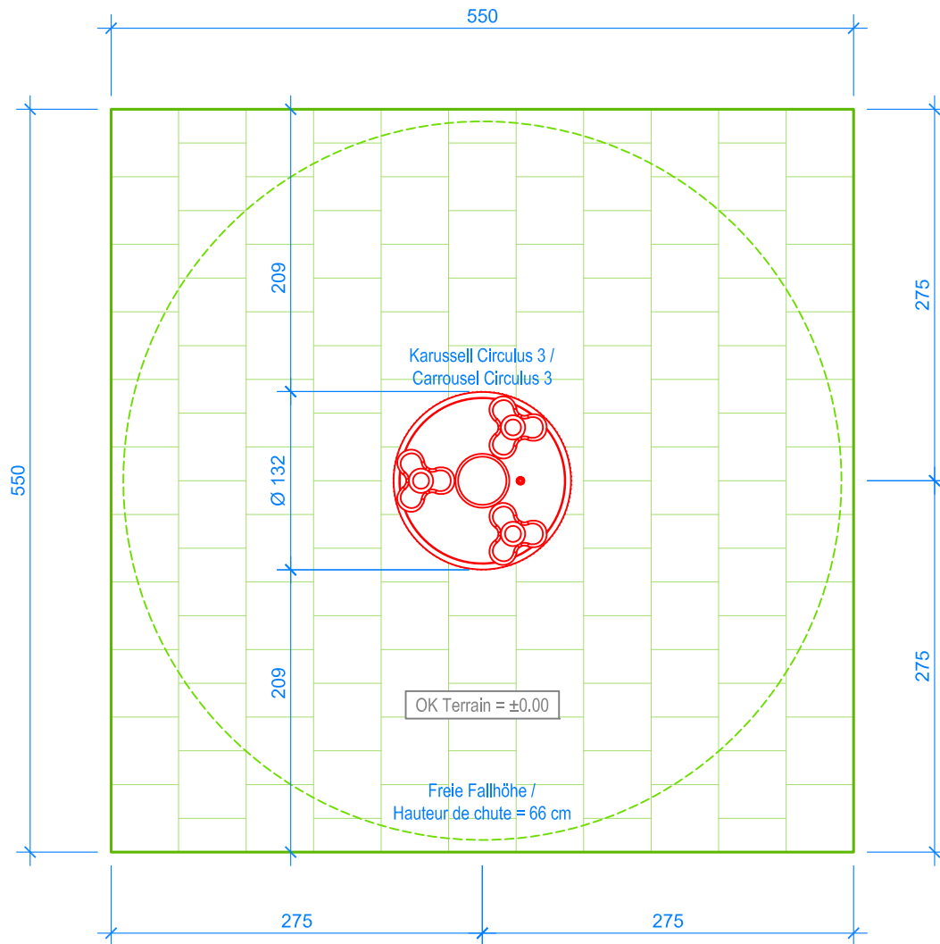
GRUNDRISS / PLAN 1:50
