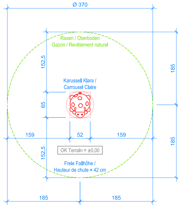
GRUNDRISS / PLAN 1:50
