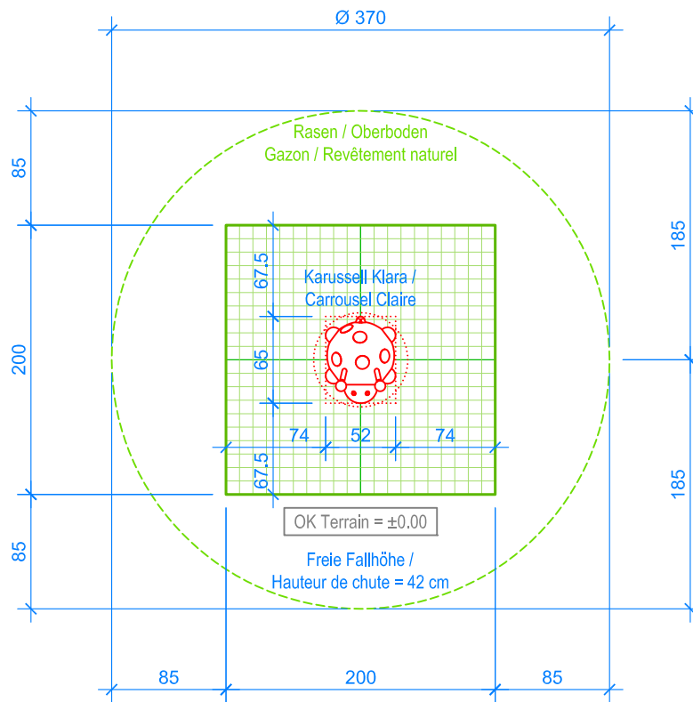
GRUNDRISS / PLAN 1:50
