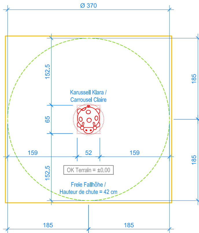
GRUNDRISS / PLAN 1:50
