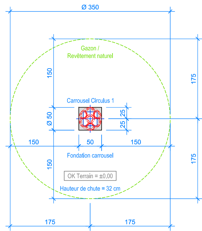
PLAN 1:50
