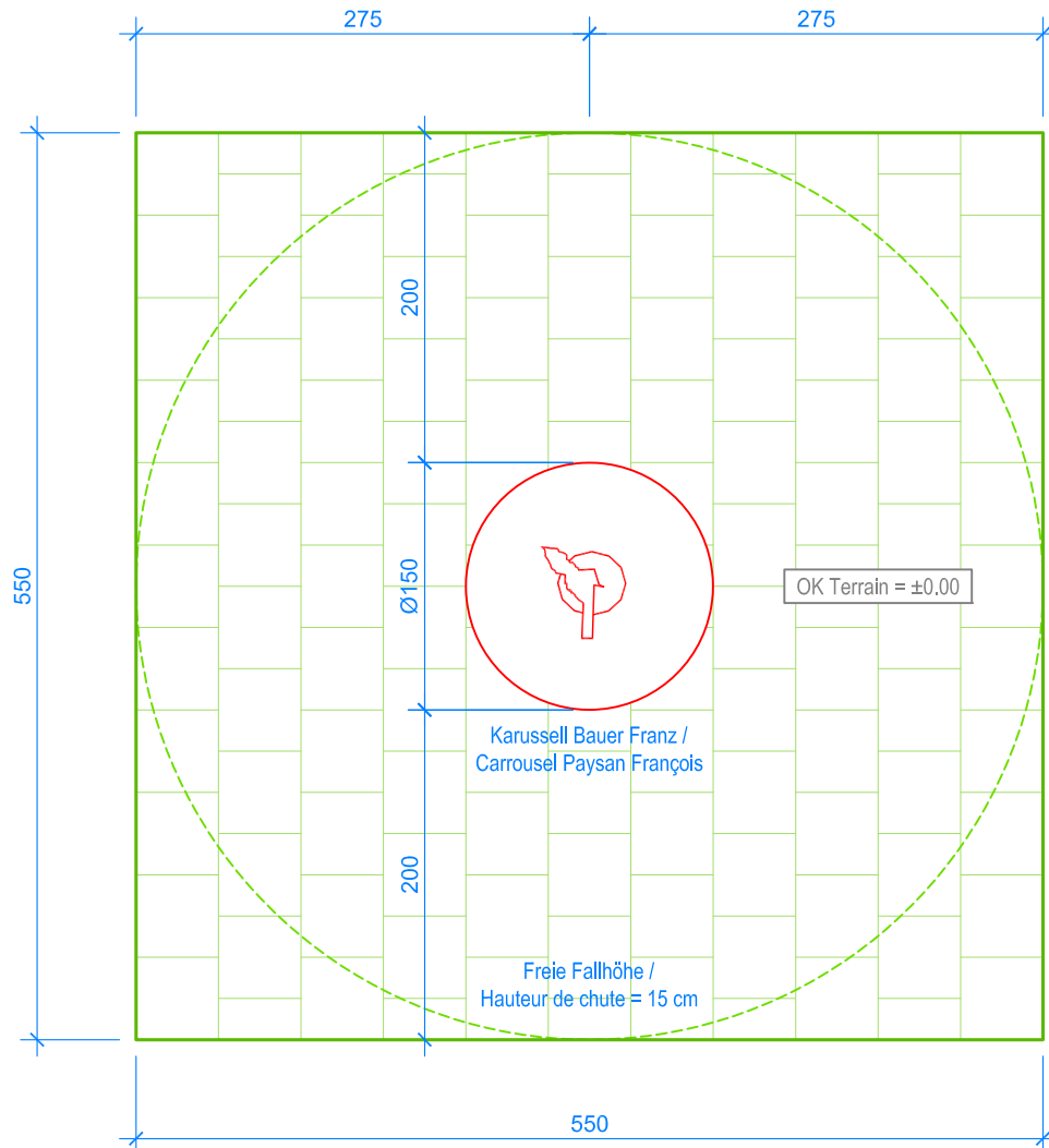
GRUNDRISS / PLAN 1:50
