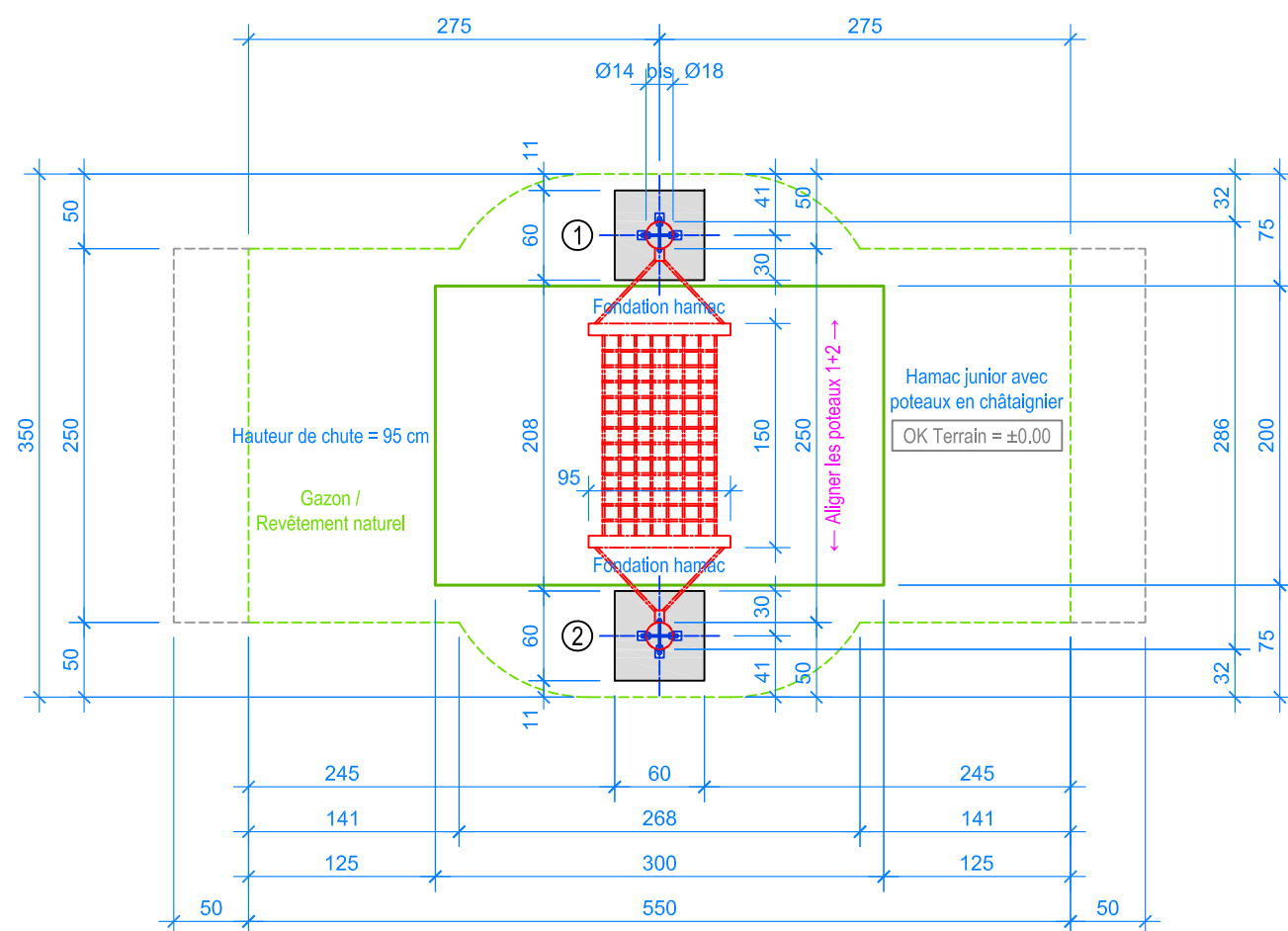
PLAN 1:50
