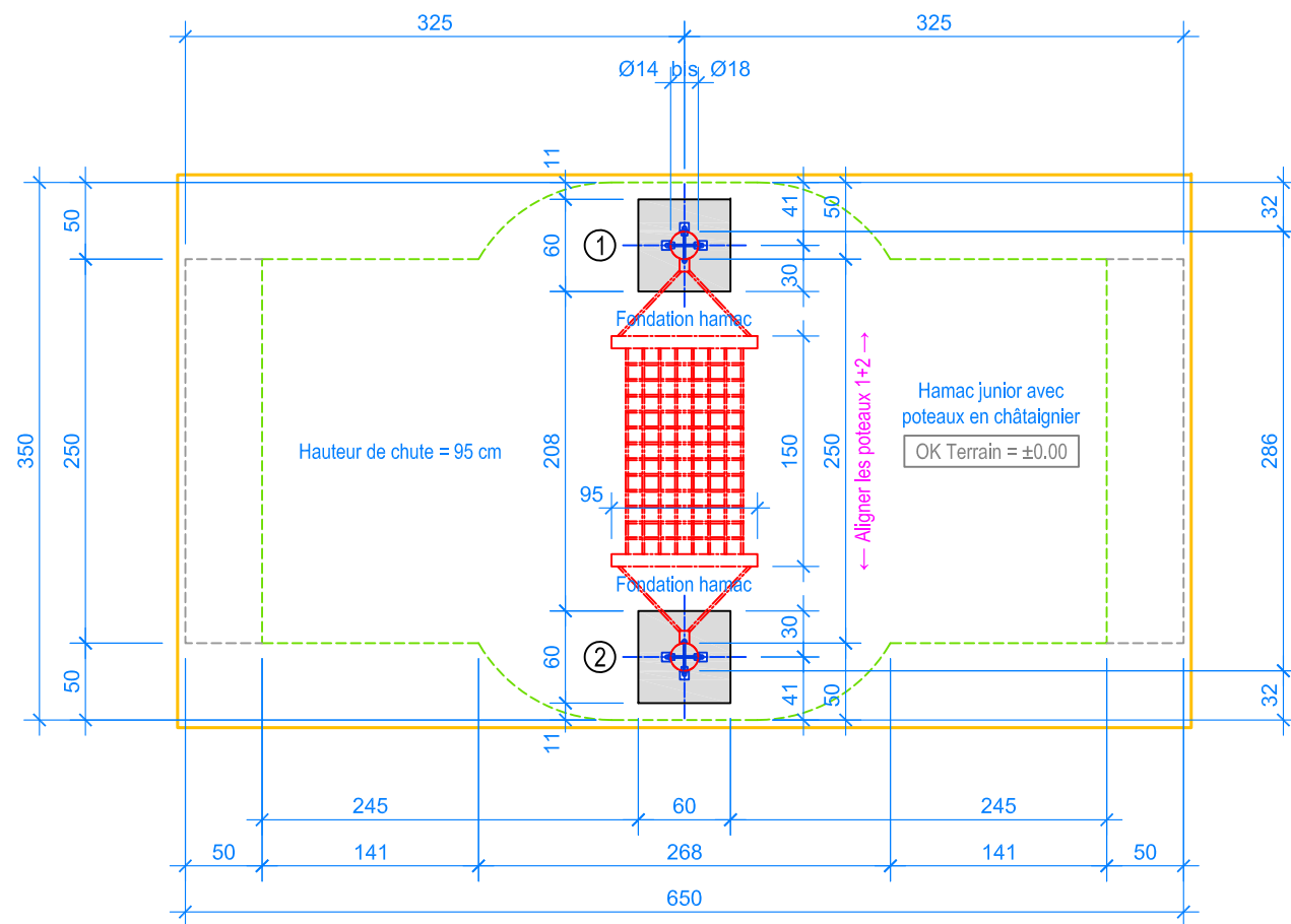
PLAN 1:50
