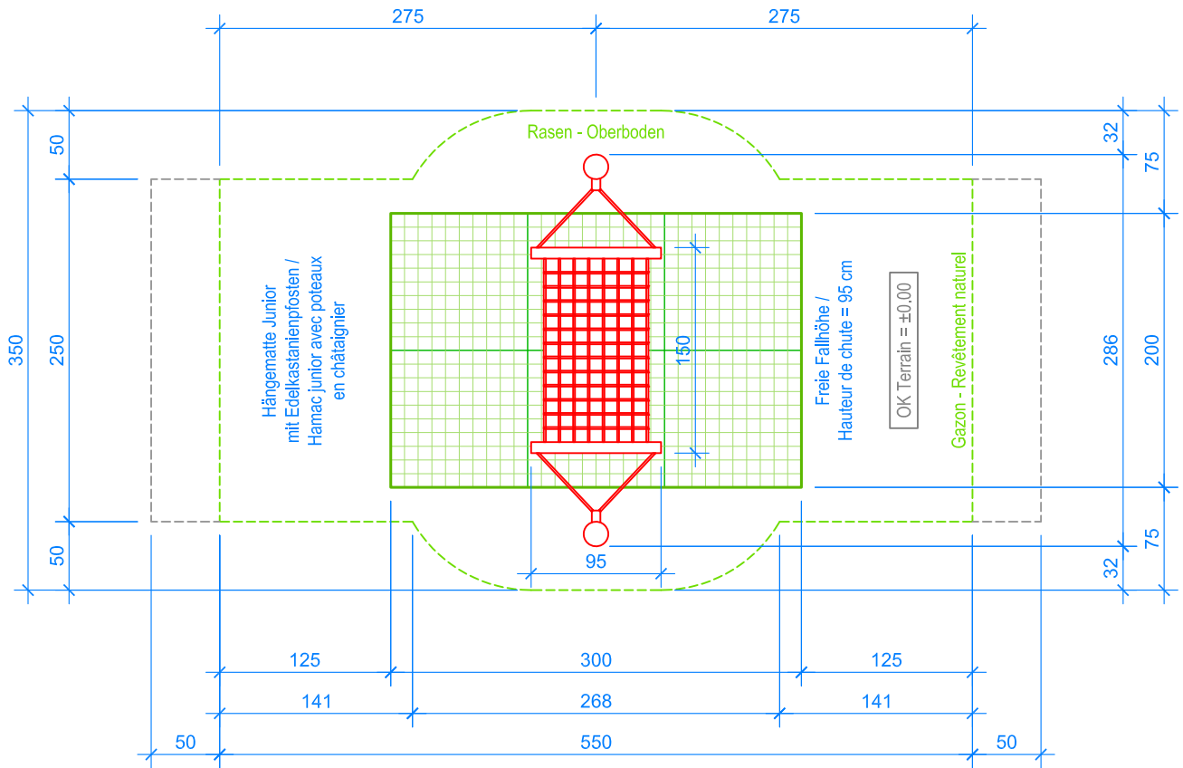
GRUNDRISS / PLAN 1:50
