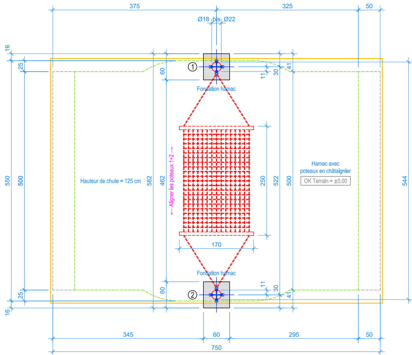
PLAN 1:50
