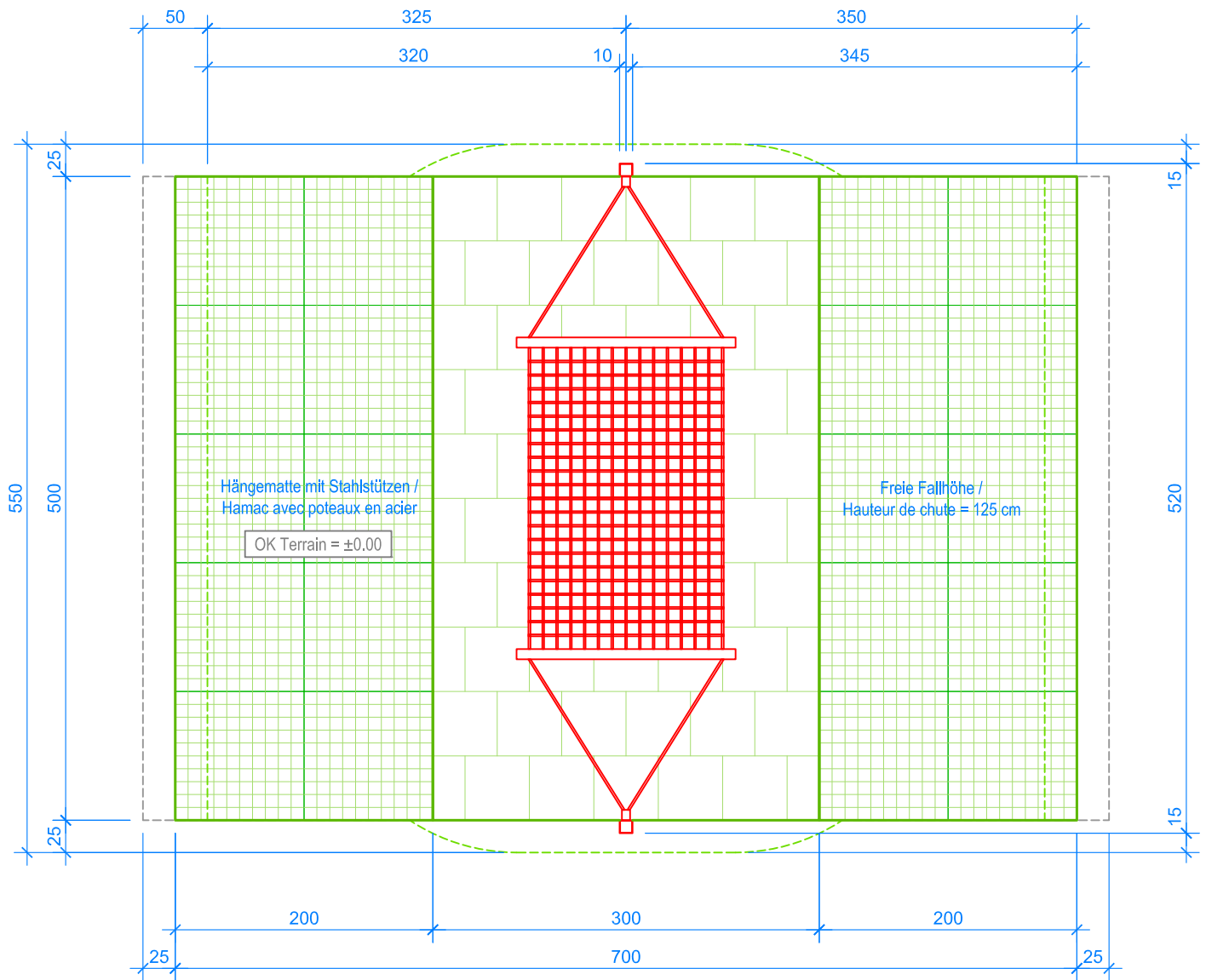
GRUNDRISS / PLAN 1:50
