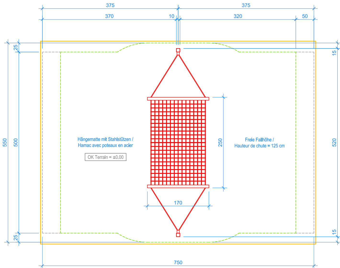
GRUNDRISS / PLAN 1:50
