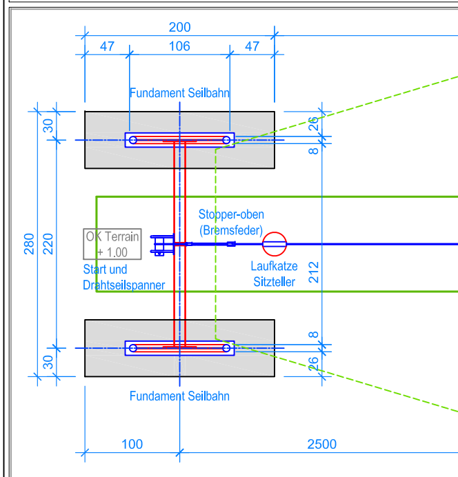
GRUNDRISS 1:55
