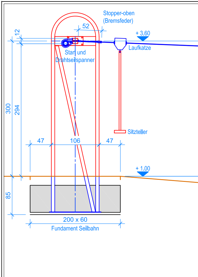
LÄNGSSCHNITT 1:55
