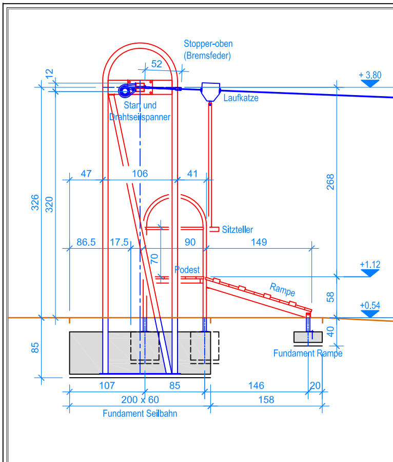
LÄNGSSCHNITT 1:55
