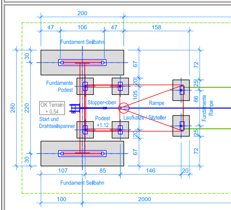
GRUNDRISS 1:55
