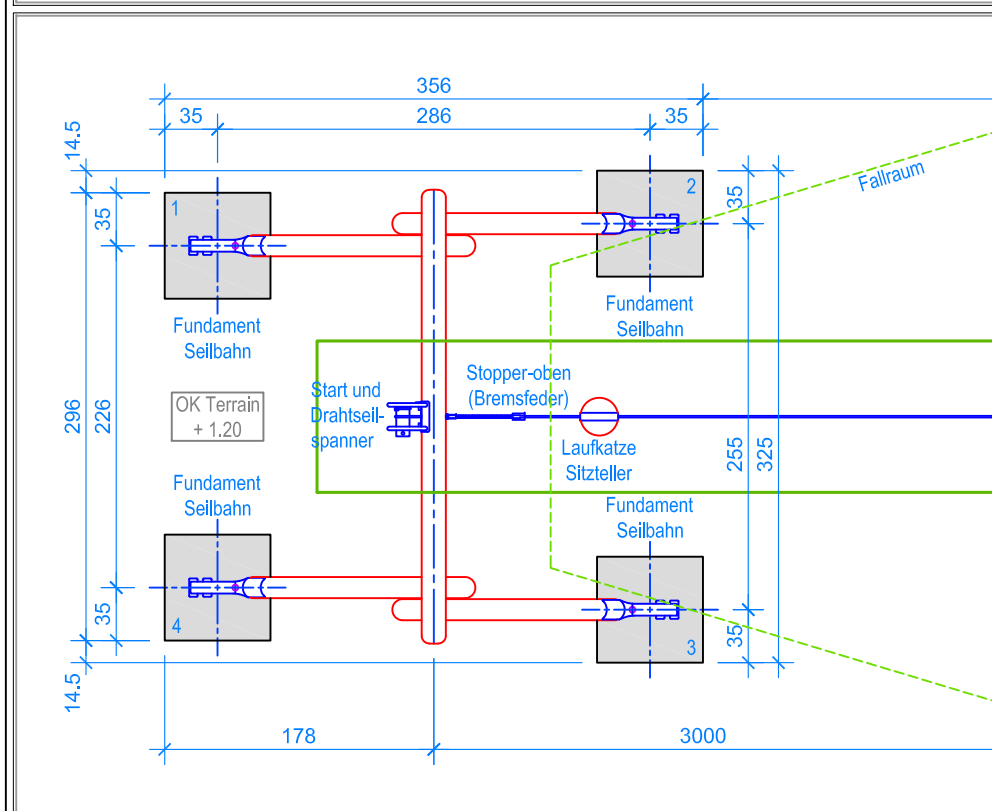
GRUNDRISS 1:50
