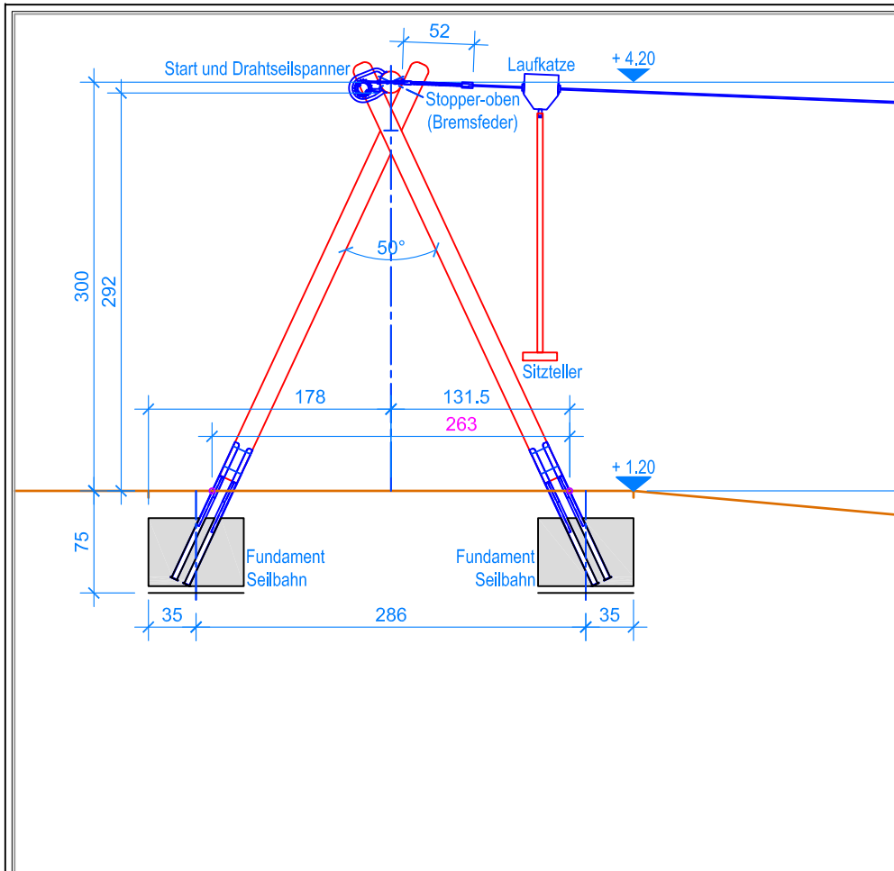
LÄNGSSCHNITT 1:50
