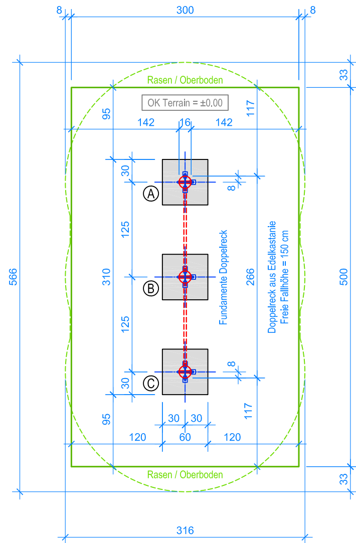
GRUNDRISS 1:50
