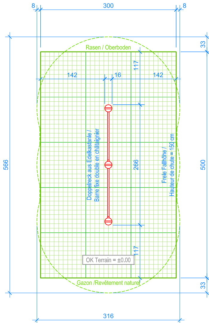
GRUNDRISS / PLAN 1:50
