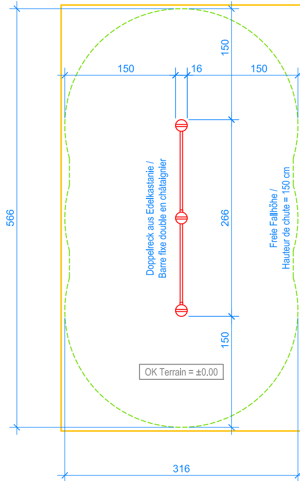
GRUNDRISS / PLAN 1:50
