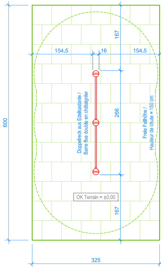
GRUNDRISS / PLAN 1:50
