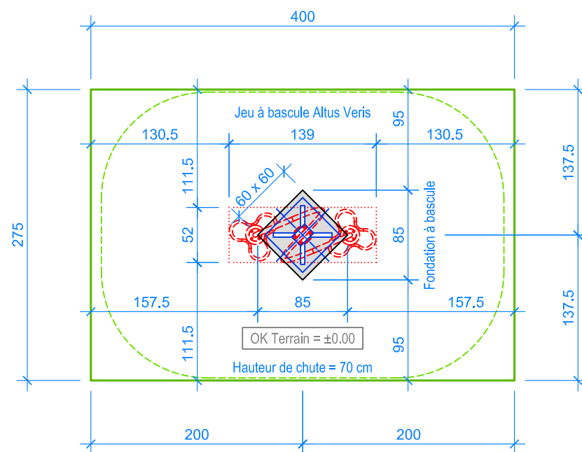
PLAN 1:50
