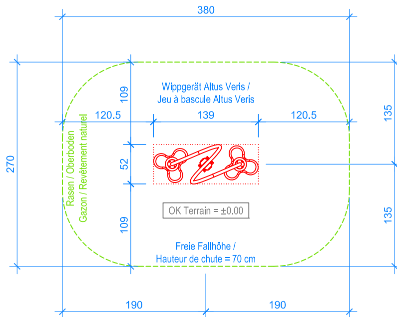
GRUNDRISS / PLAN 1:50
