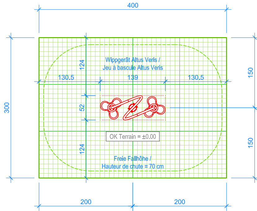
GRUNDRISS / PLAN 1:50
