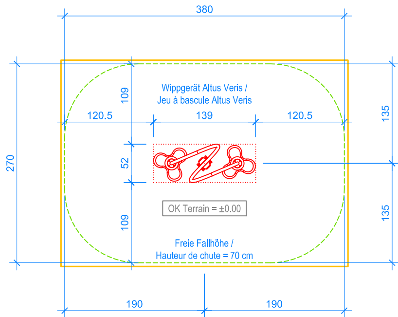
GRUNDRISS / PLAN 1:50
