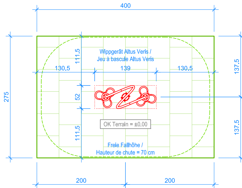
GRUNDRISS / PLAN 1:50
